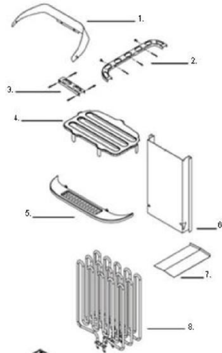
Abb. 10 Ersatzteile Fig. 10 Spare parts
